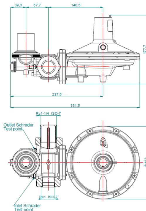
Fig. 4 – Dimensões externas (com OPSO)
