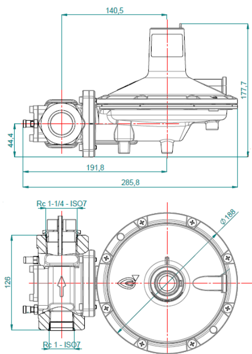
Fig. 3 – Dimensões externas (s/ OPSO)
