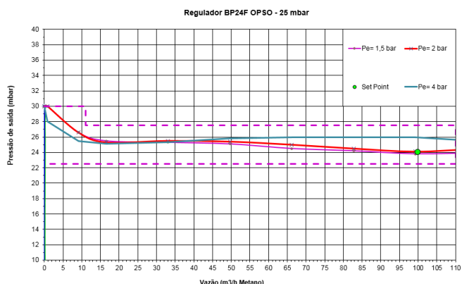
Gráfico 1 – Pressão de saída em 25 mbar
