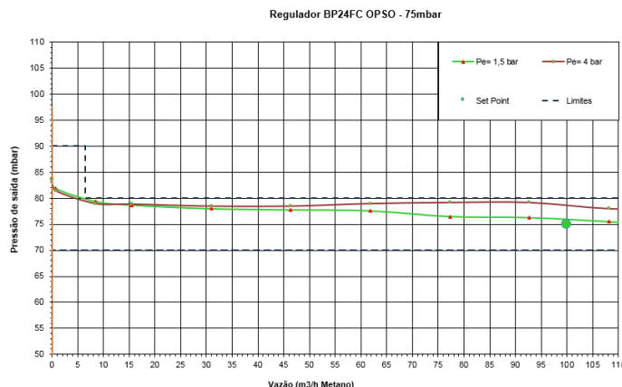
Gráfico 2– Pressão de saída em 75 mbar
